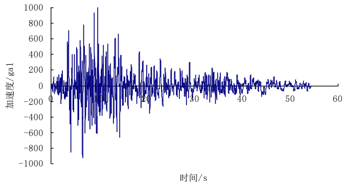
图 3 Taft 波波形 (放大至峰值为 1000gal)
